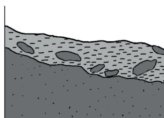
3. Seconde phase de sédimentation. Remobilisation d'éléments de la roche A. Formation de la roche B.
