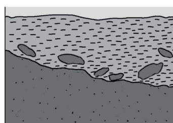
3. Seconde phase de sédimentation. Remobilisation d'éléments de la roche A. Formation de la roche B.
