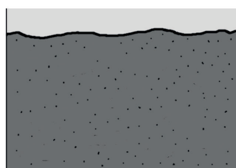
1. Première phase de sédimentation. Formation de la roche A.
