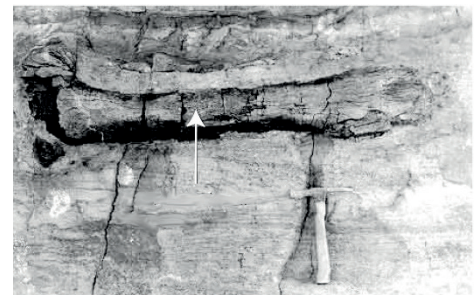
Photographie du fossile d'Hadrosaure en place dans les roches de la formation Ojo Alamo.
